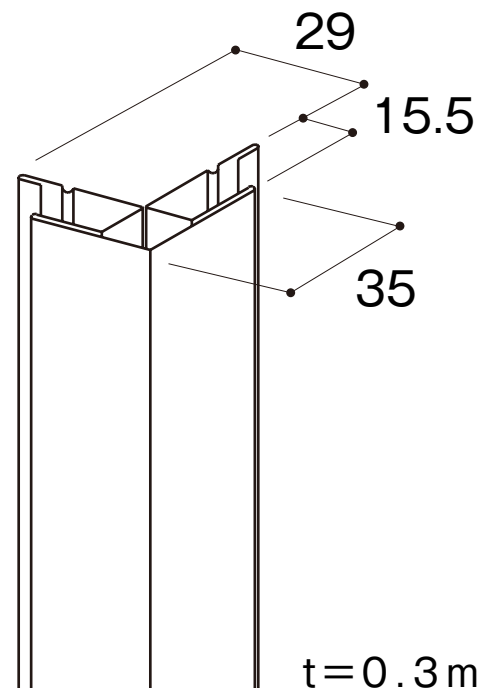
差込み出隅
