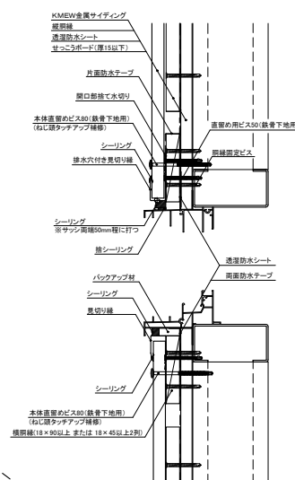
3 縦断面(排水穴付き見切り縁仕様)
