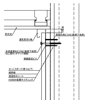
2 通気見切り縁 納まり
