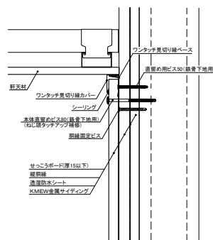
3 ワンタッチ見切り縁 納まり
