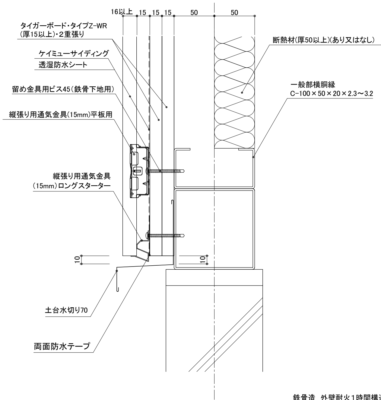
鉄骨造 外壁耐火1時間構造仕様1(内装材【指定なし】) 縦張り・通気金具留め 土台部納まり参考図
