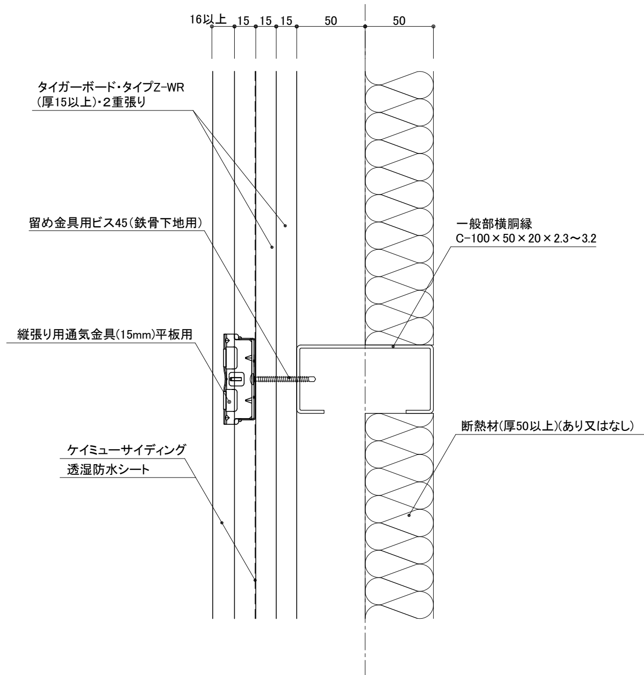
鉄骨造 外壁耐火1時間構造仕様1(内装材【指定なし】) 縦張り・通気金具留め 一般部納まり参考図
