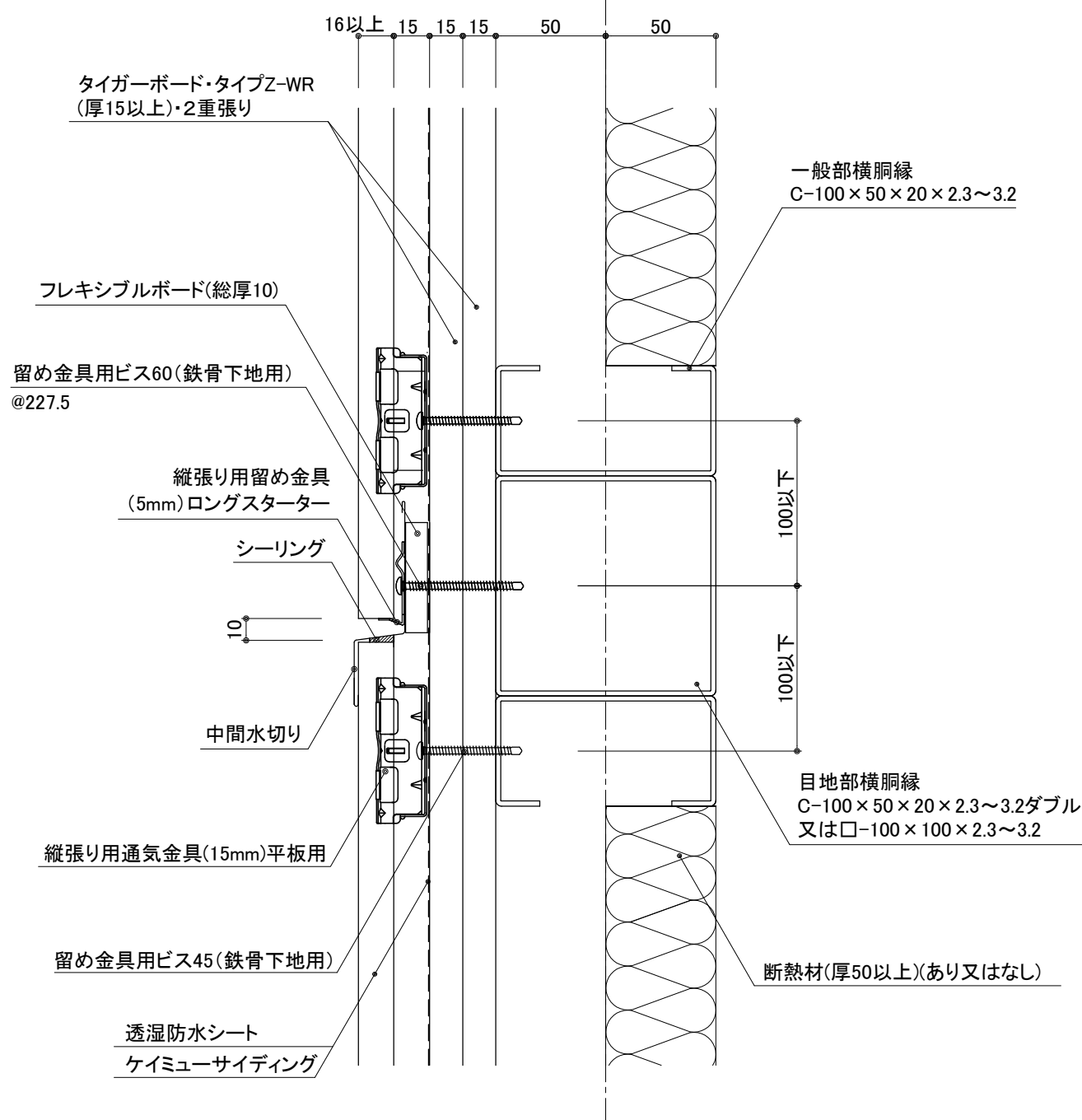
鉄骨造 外壁耐火1時間構造仕様1(内装材【指定なし】) 縦張り・通気金具留め 横目地部納まり参考図
