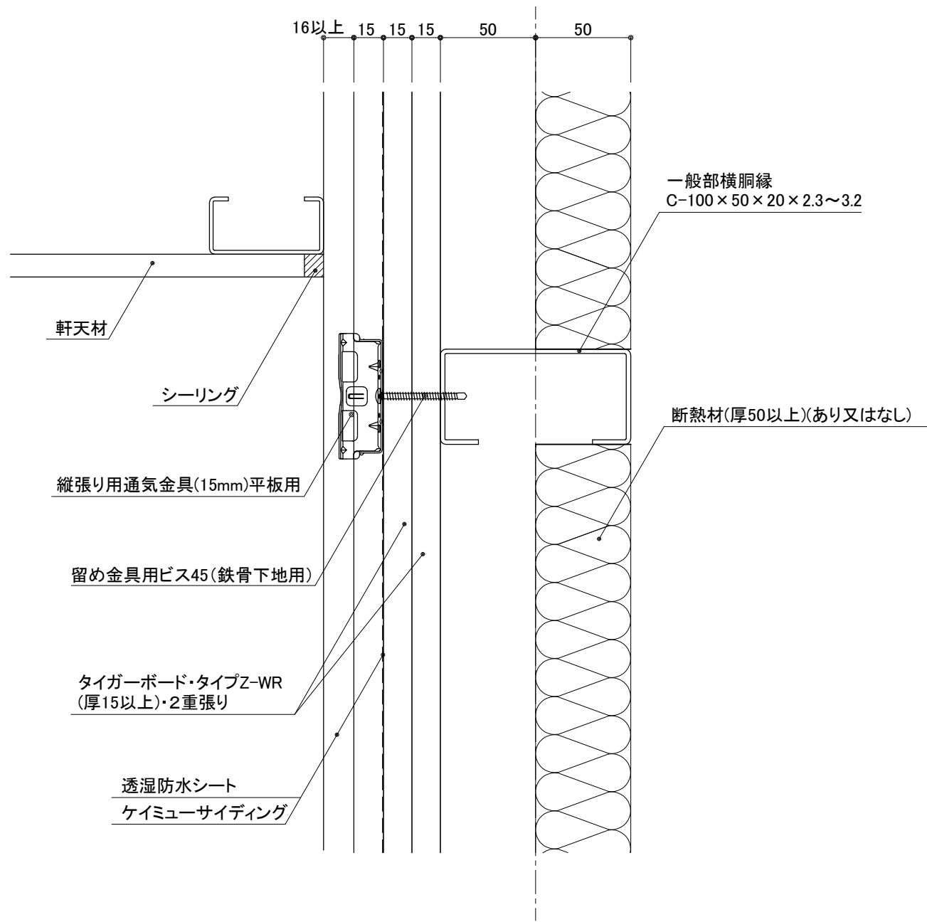
鉄骨造 外壁耐火1時間構造仕様1(内装材【指定なし】) 縦張り・通気金具留め 軒天部納まり参考図
