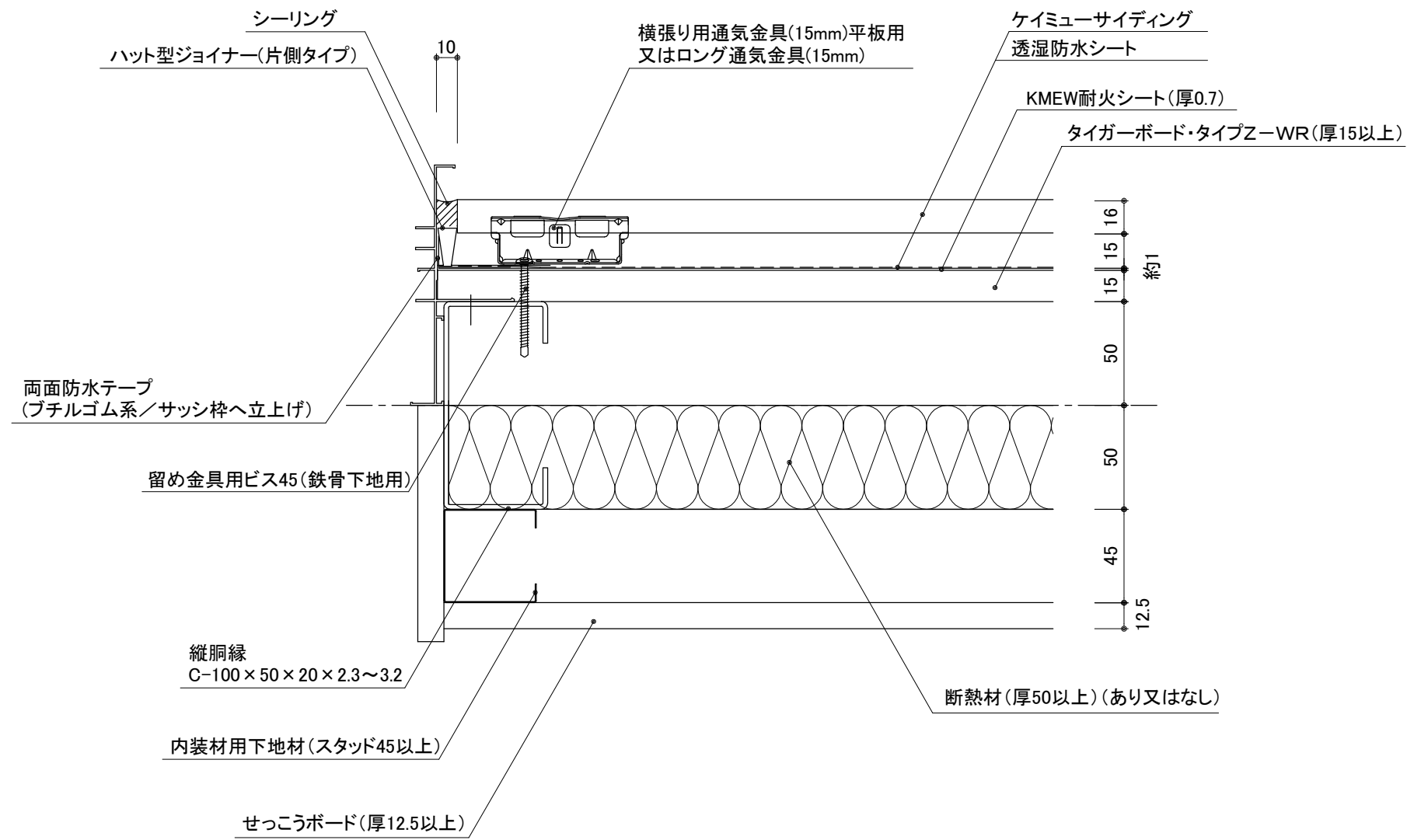
鉄骨造 外壁耐火1時間構造仕様2(内装材【指定あり】・耐火シート仕様) 横張り・通気金具留め 開口部(横断面)半外サッシ納まり参考図
