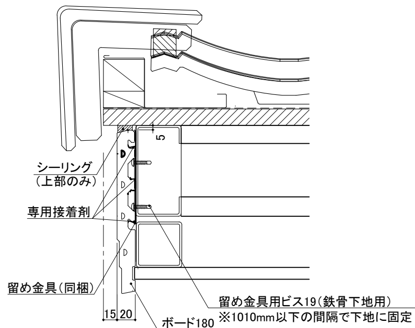
鉄骨造 破風 (ウォールライン ボード180) 納まり参考図
