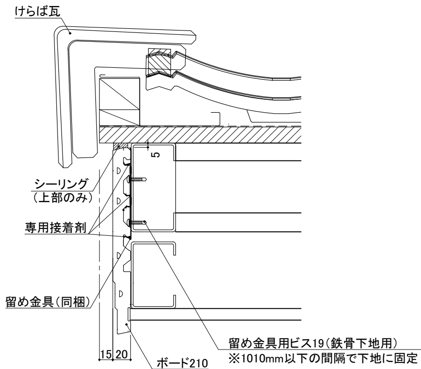
鉄骨造 破風 (ウォールライン ボード210) 納まり参考図
