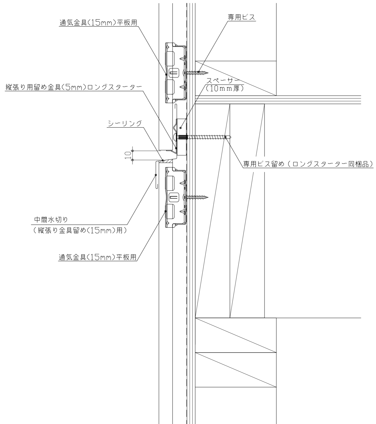
木造・縦張り・通気金具留め 横目地部(中間水切り)納まり参考図
