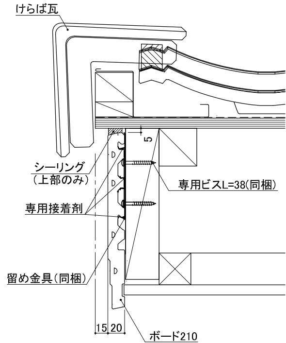
木造 破風(ウォールライン ボード210)納まり参考図
