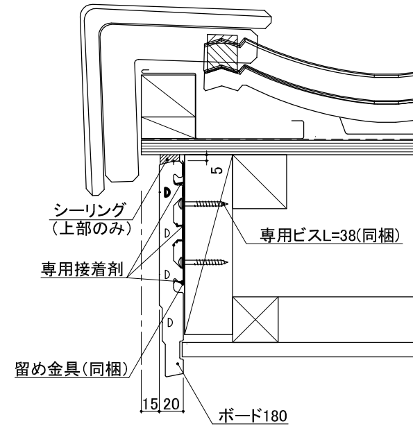
木造 破風(ウォールライン ボード180)納まり参考図
