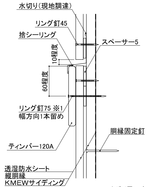
木造(雪の多い地域)・横張り・5mm金具留め 幕板(ウォールライン ティンバー120A)納まり参考図
