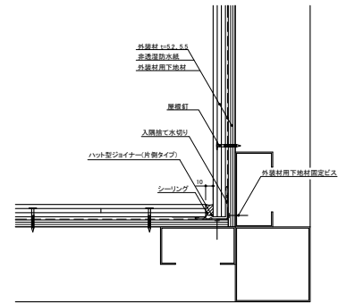
1 シーリング 納まり
