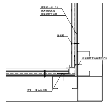
3 スマート差込み入隅 納まり
