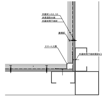
2 スマート入隅 納まり
