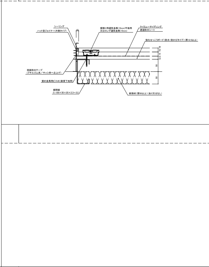
4 横断面(半外サッシ)
