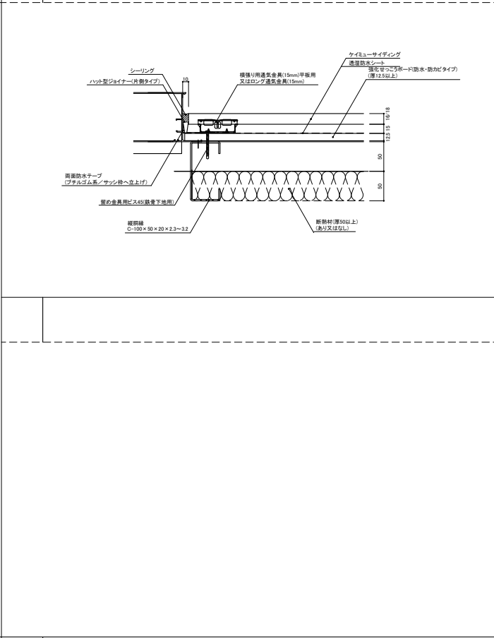
6 横断面(外見切りサッシ)
