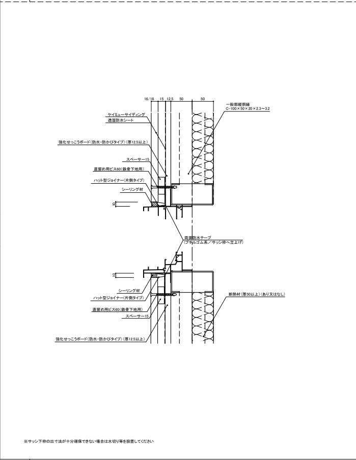
3 縦断面(半外サッシ)
