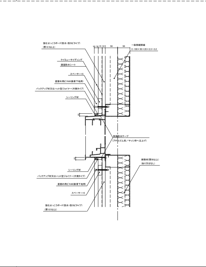
5 縦断面(外見切りサッシ)
