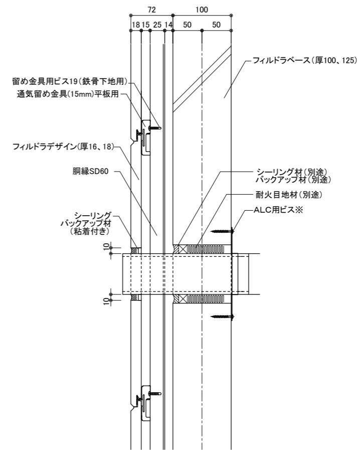
断面図
