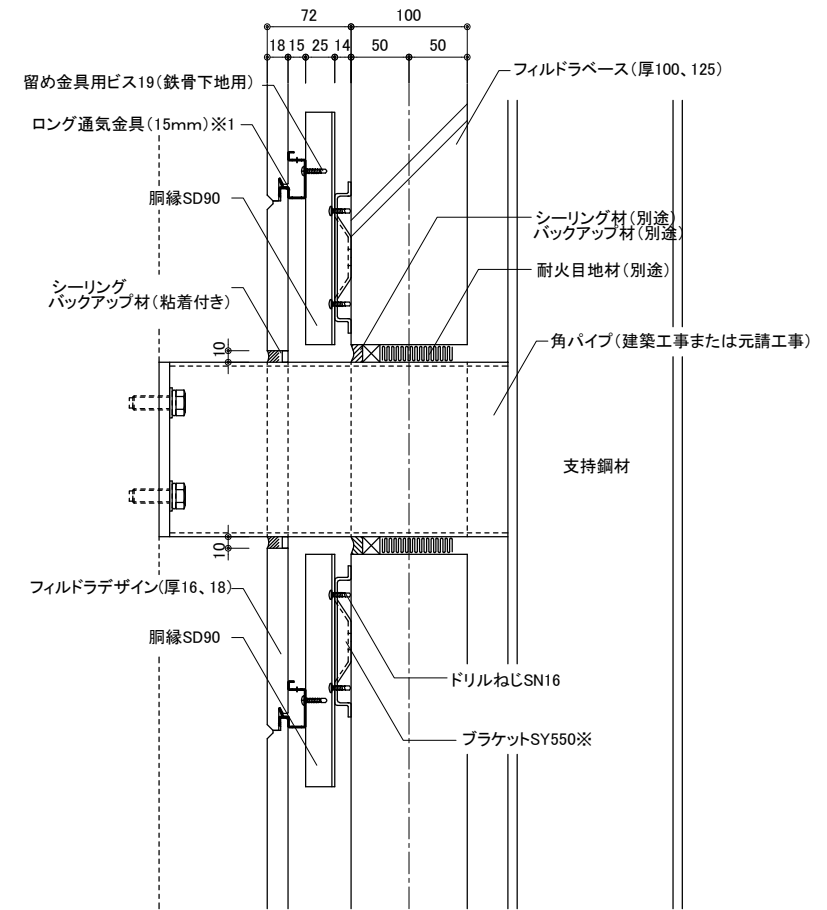
断面図
