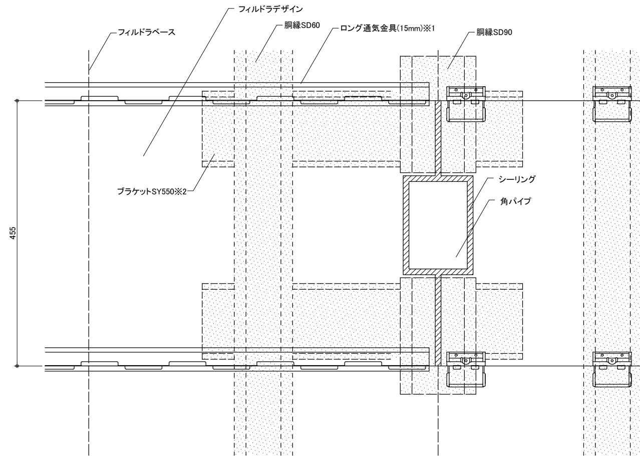
胴縁・フィルドラ・デザイン割付け参考図
