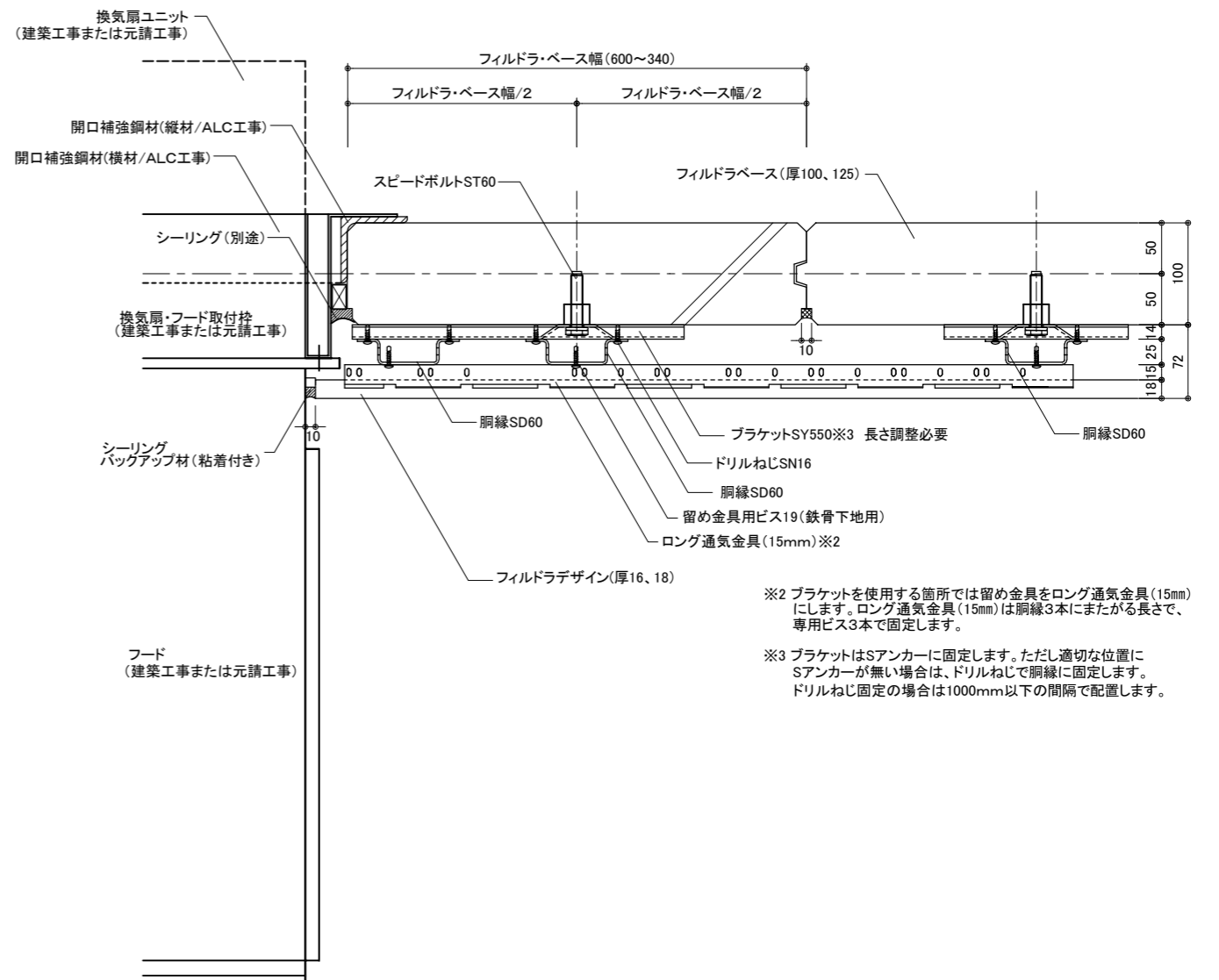
平面図
