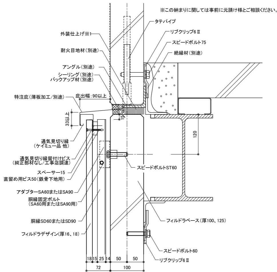
断面図(フィルドラ・デザイン上部終端部)
