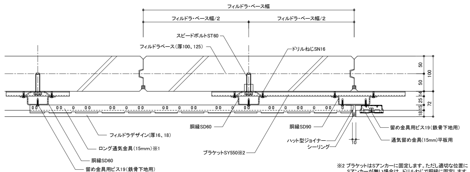
平面図(縦目地位置調整)
