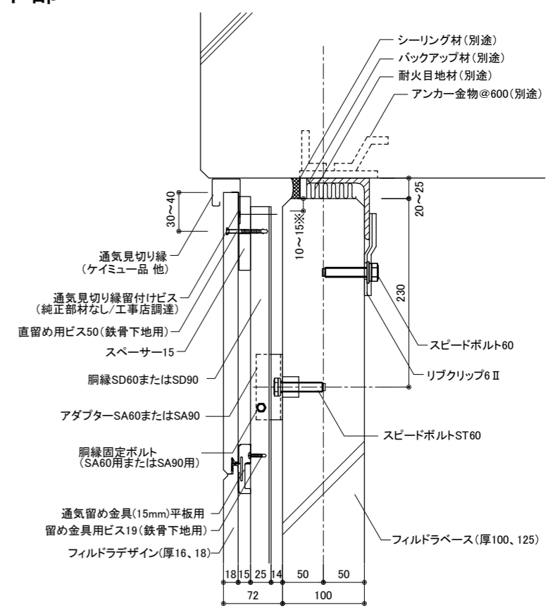
断面図
