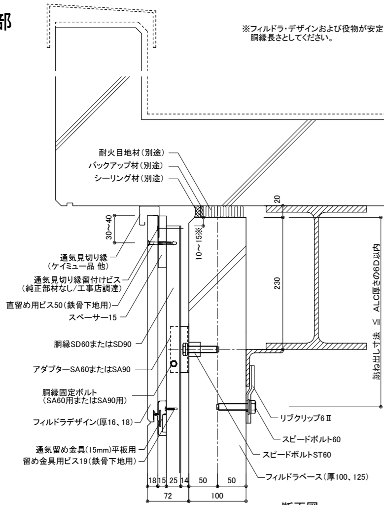
断面図
