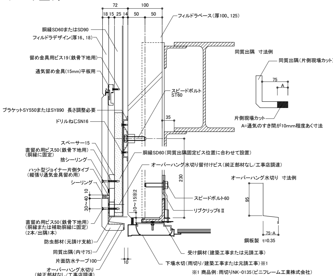
断面図
