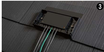
中部材を取り付け配線ケーブルを引込みます。配線カバーを取付け上部材を取付けます。
