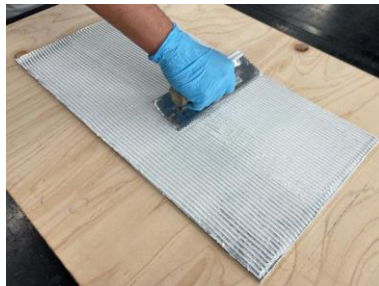
SOLIDO裏面への接着剤塗布 (くし目3mm)
