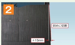
2 本体を、勝ち負けで突付けて納めます。まず、負け側の面を施工します。本体上端は捨水切の角部、本体下端は角部より+15mmの位置で、斜めに切断して固定します。
