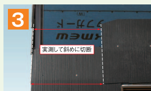
3 勝ち側の面は、負け側の本体木口を隠すように寸法を実測し、斜めに切断して固定します。
